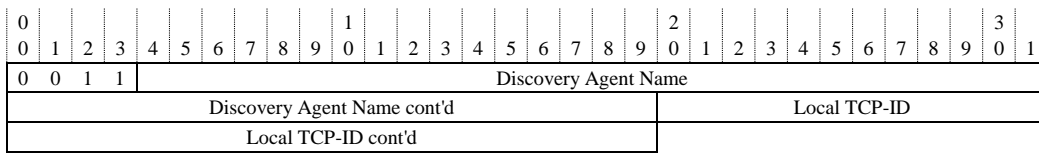
Figure 6/G.7714.1/Y.1705.1 – DA DCN Name Message format
