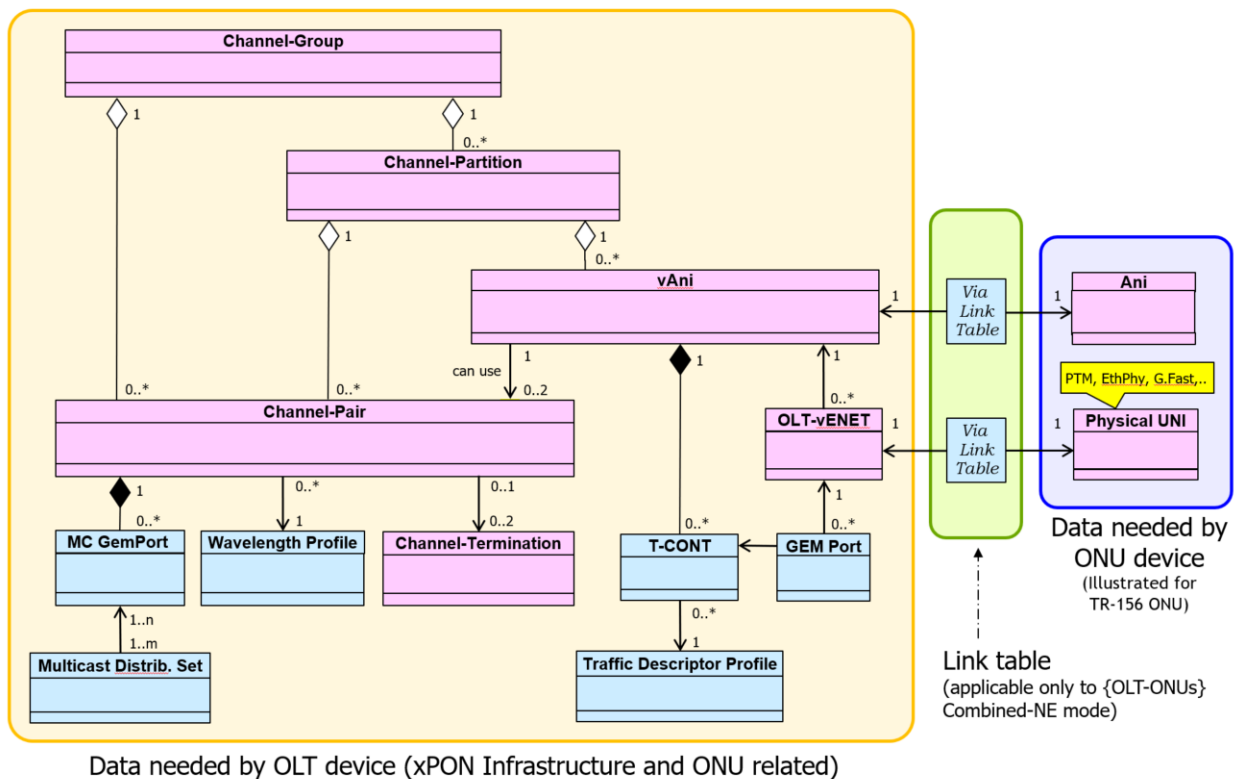
Figure 6-1/Figure 29 – xPON YANG UML Model
