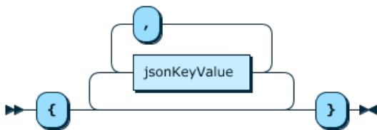
Figure 12.17 jsonDoc
